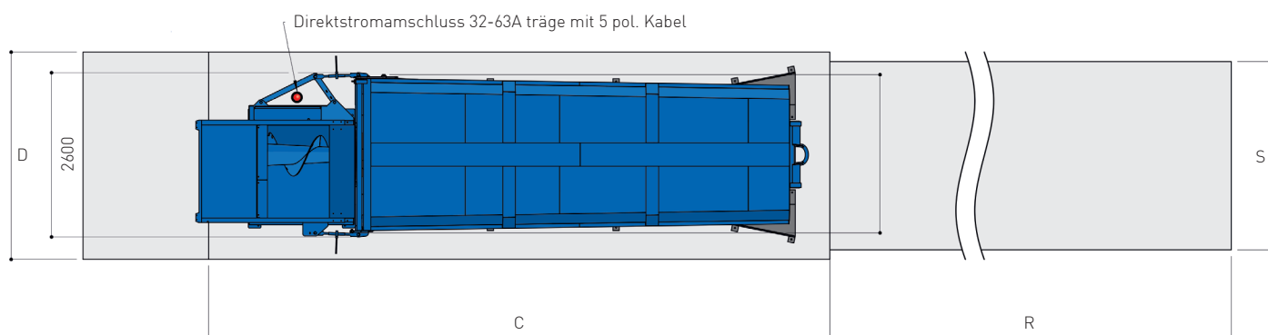
GRUNDRISS
