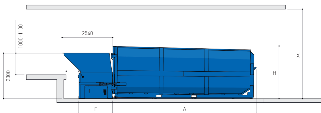
SEITENANSICHT
