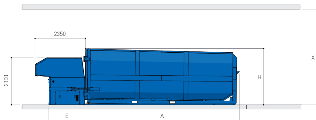
SEITENANSICHT
