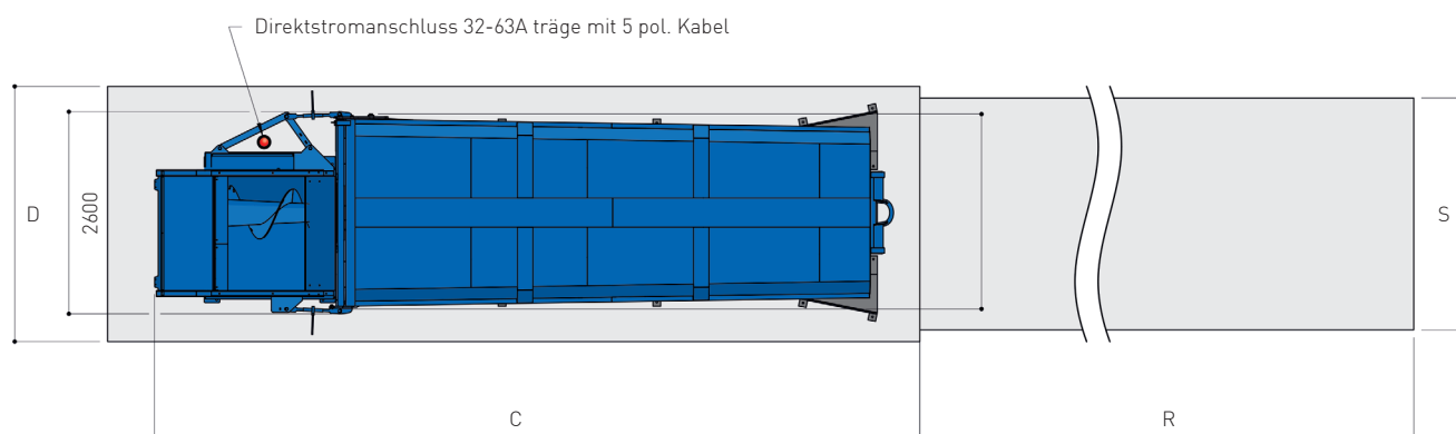
GRUNDRISS
