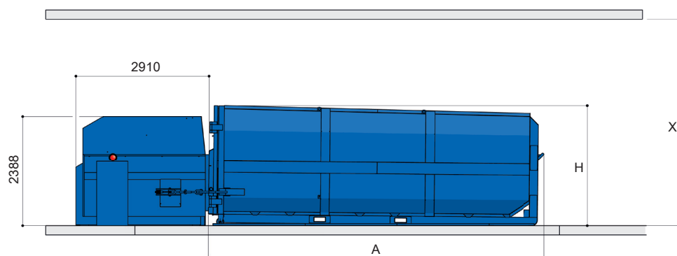
SEITENANSICHT
