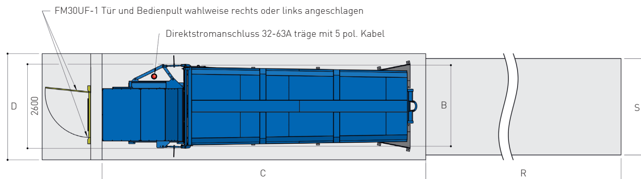
GRUNDRISS
