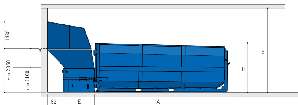
SEITENANSICHT
