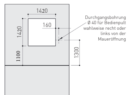
INNENANSICHT
