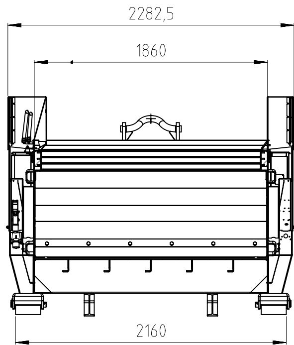
SNITT B-B
