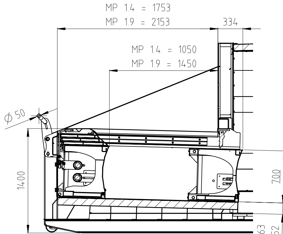
SNITT A-A
